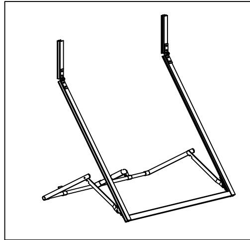
Telaio a sporgere con leva centrale: art.6070 per profili da 7.5-9mm. art.6071 per profili da 12-14mm.
